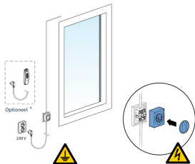
Motor links (van buitenaf gezien)
