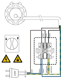
Motor links (van buitenaf gezien)
