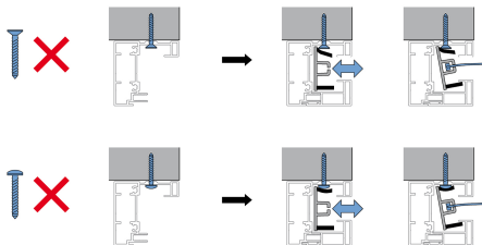
fig. 1.6 Onjuiste montage
