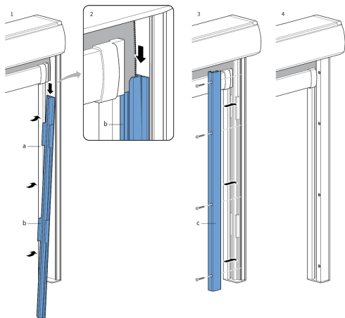
fig. 1.8 Monteren geleider
