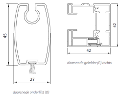
doorsnede onderlijst (O)
