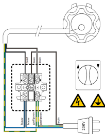
Motor rechts (van buitenaf gezien)
