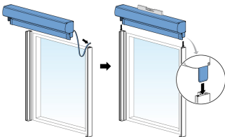
Fig. 1.7 Plaatsen screenkap
